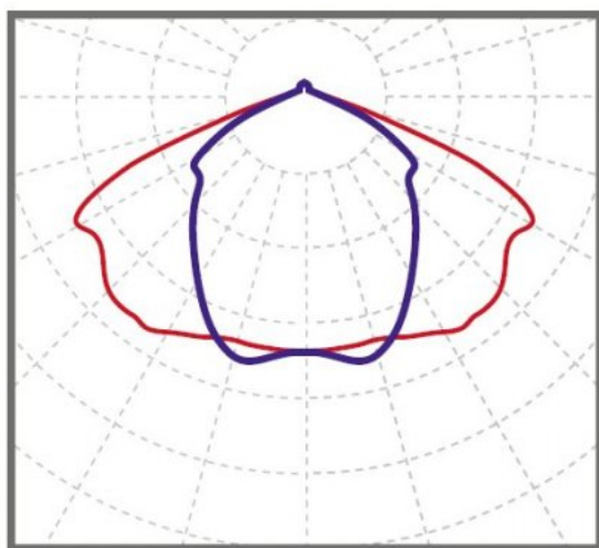
полуширокая осевая КСС 140°x95°
